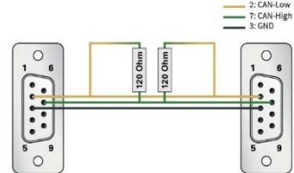
PCAN-Cable 2
